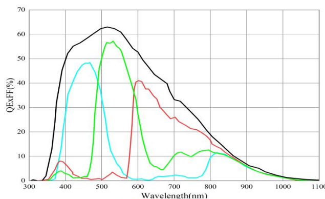
相机光谱响应曲线
